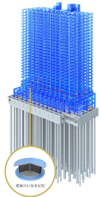
免震構造概念図
